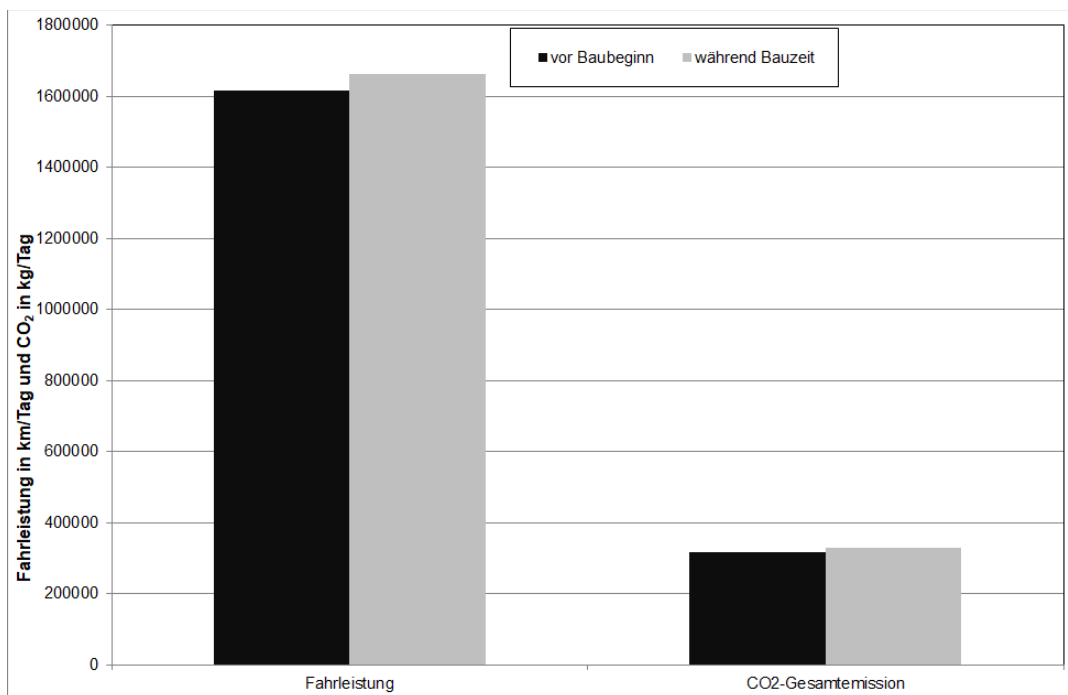
Abb. A1: Summe der klimarelevanten CO 2 -Emission für Straßenabschnitte im Betrachtungsgebiet
