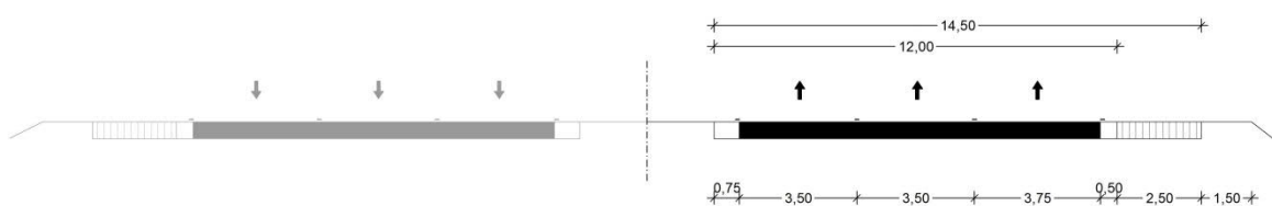
Abbildung 1. Querschnittszusammensetzung RQ 36
